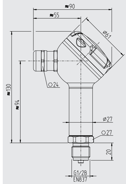
Custodia da campo Pressacavo filettato regolabile
