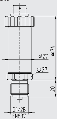
Connettore a baionetta MIL-DTL-26482 (6 pin) regolabile
