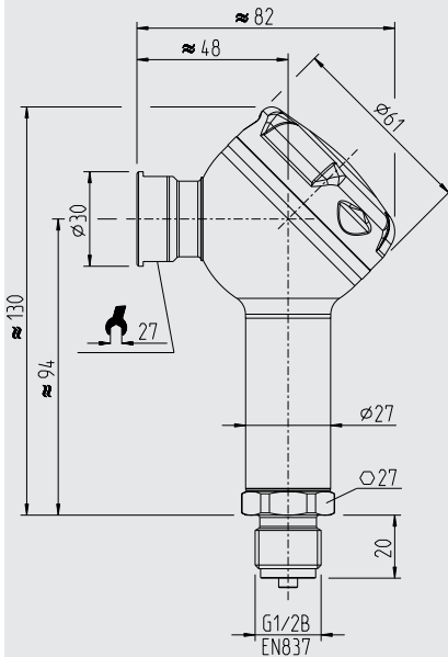
Custodia da campo Conduit M20 x 1,5-I regolabile
