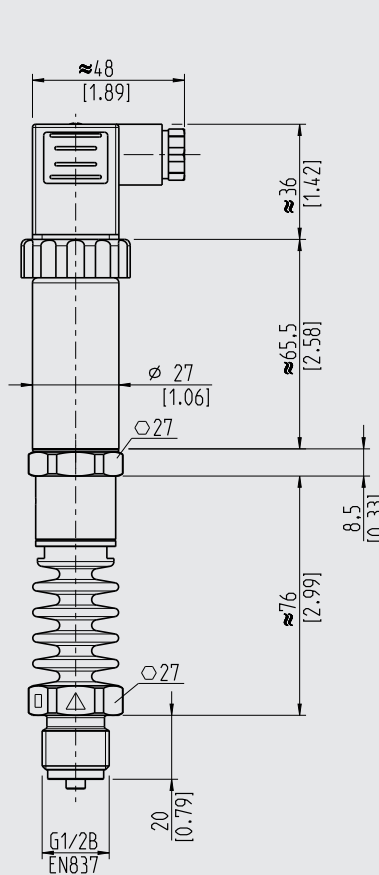
IS-3 per temperature del fluido opzionali -40 ... +150 °C [-40 ... 302 °F] e -40 ... +200 °C [-40 ... +392 °F]
