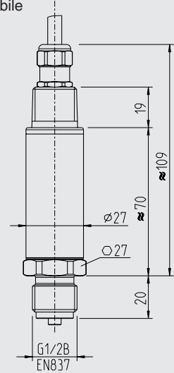
Uscita cavo IP68 Pressacavo, conduit 1/2 NPT non regolabile
