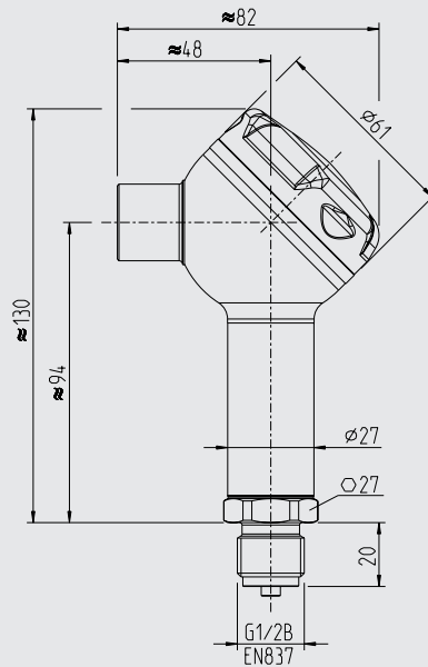
IS-3 per temperature del fluido opzionali -40 ... +150 °C [-40 ... 302 °F] e -40 ... +200 °C [-40 ... +392 °F]
