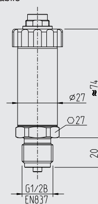
Connettore circolare M16 x 0,75 IEC 61076-2-106 (5 pin) regolabile
