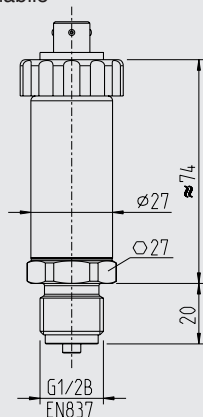
Connettore a baionetta MIL-DTL-26482 (4 pin) regolabile
