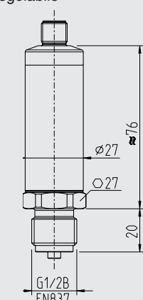
Connettore circolare M12 x 1 IEC 61076-2-101 A-COD (4 pin) non regolabile
